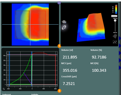
3D 焊点测量
