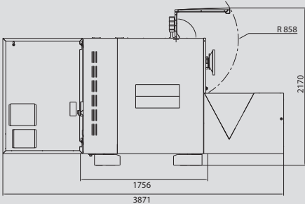
侧视图
