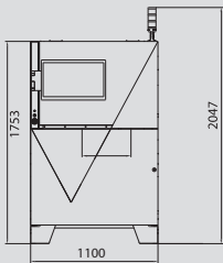
正视图
