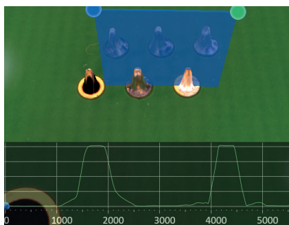
THT上的高度剖面
