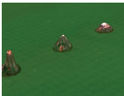
对引脚长度执行可靠的3D检测
