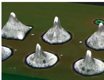
THT焊接点的3D质量控制
